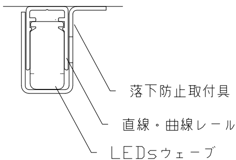
参考 嵌合図
